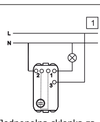
Jednopolna sklopka za kupatilo Single-pole switch with zero contact
