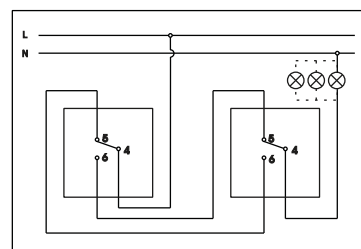
Naizmenična sklopka Two-way switch
