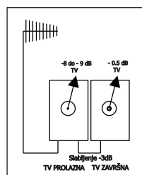
TV priključnica 2M prolazno završna TV aerial socket 2M feed through & terminal
