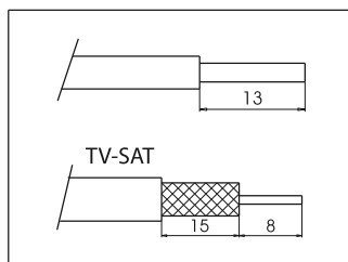
Kombo - Blankiranje provodnika za TV priključnice Kombo - Removing isolation for TV aerial sockets
