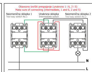
Povezivanje unakrsne sklopke Wiring of intermediate switch
