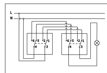
Dvopolna naizmenična sklopka Two-way double-pole switch
