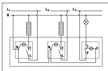
Vertikalna sklopka za kupatilo Vertical bathroom switch
