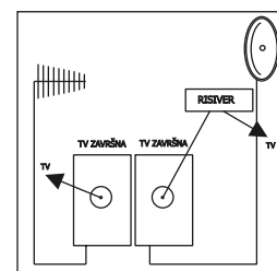
TV priključnica 2M završna TV aerial socket 2M terminal
