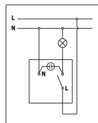
Jednopolna sklopka (KIP) Single-pole switch (KIP)
