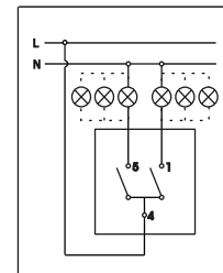
Serijska sklopka Two-circuit switch
