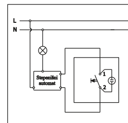
Taster svetla sa signalnom sijalicom Light push-button with pilot light
