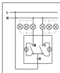
Serijska sklopka sa signalnom sijalicom Two-circuit switch with pilot lights
