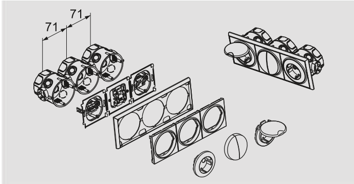
Montaža nizajuće dozne Mounting box for multiple frames - deep
