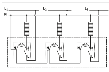
Horizontalna sklopka za kupatilo Horizontal bathroom switch
