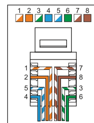
Komunikaciona Cat6 UTP Communication socket Cat6 UTP
