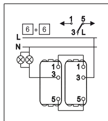
Kombo - Naizmjenična sklopka Kombo - Two-way switch - wiring
