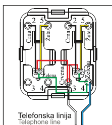
Telefonska priključnica Telephone socket
