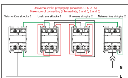
Povezivanje dve unakrsne sklopke Wiring of two intermediate switches
