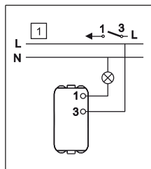
Kombo - Jednopolna sklopka Kombo - Single-pole switch - wiring
