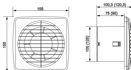
Ventilator za kupatilo-Fluent 100 Bathroom fan-Fluent 100
