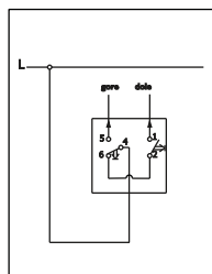
Taster za roletne Blind control button
