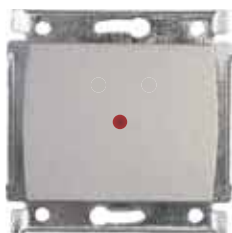
Jednopolna sklopka sa signalnom sijalicom Single-pole switch with pilot light 10AX/250V; IP 20
