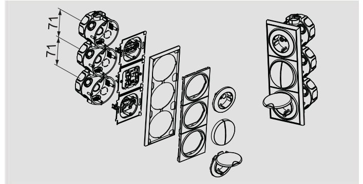
Montaža vertikalnog nizajućeg okvira Mounting of vertical decorative frames
