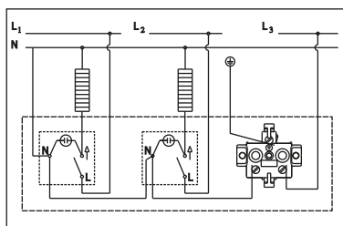
Vertikalna sklopka za kupatilo sa dvopolnom priključnicom Vertical bathroom switch with two-pole socket-outlet
