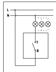
Jednopolna sklopka Single-pole switch
