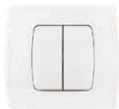
Serijska sklopka Two-circuit switch 10AX/250V; IP 20
