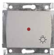
Taster svetla sa signalnom sijalicom Light push-button with pilot light 10AX/250V; IP 20
