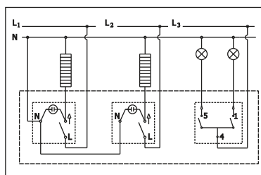
Vertikalna sklopka za kupatilo sa serijskom sklopkom Vertical bathroom switch with two-circuit switch
