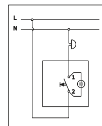
Taster sa signalnom sijalicom Push-button with pilot light
