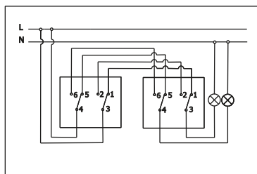
Dvostruka naizmenična sklopka Double two-way switch
