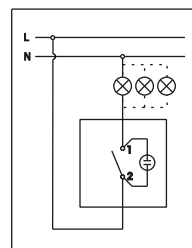
Jednopolna sklopka sa signalnom sijalicom Single-pole switch with pilot light
