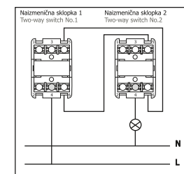
Povezivanje dve naizmenične sklopke Wiring of two-way switches
