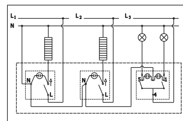
Vertikalna sklopka za kupatilo sa serijskom sklopkom i signalnim sijalicama Vertical bathroom switch with two-circuit switch and pilot lights
