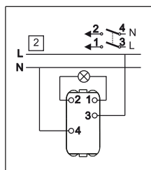
Kombo - Dvopolna sklopka Kombo - Double-pole switch - wiring
